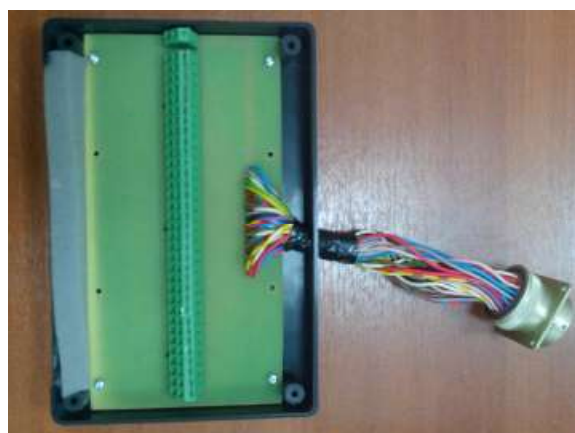
Рисунок 5 - Блок БТП
