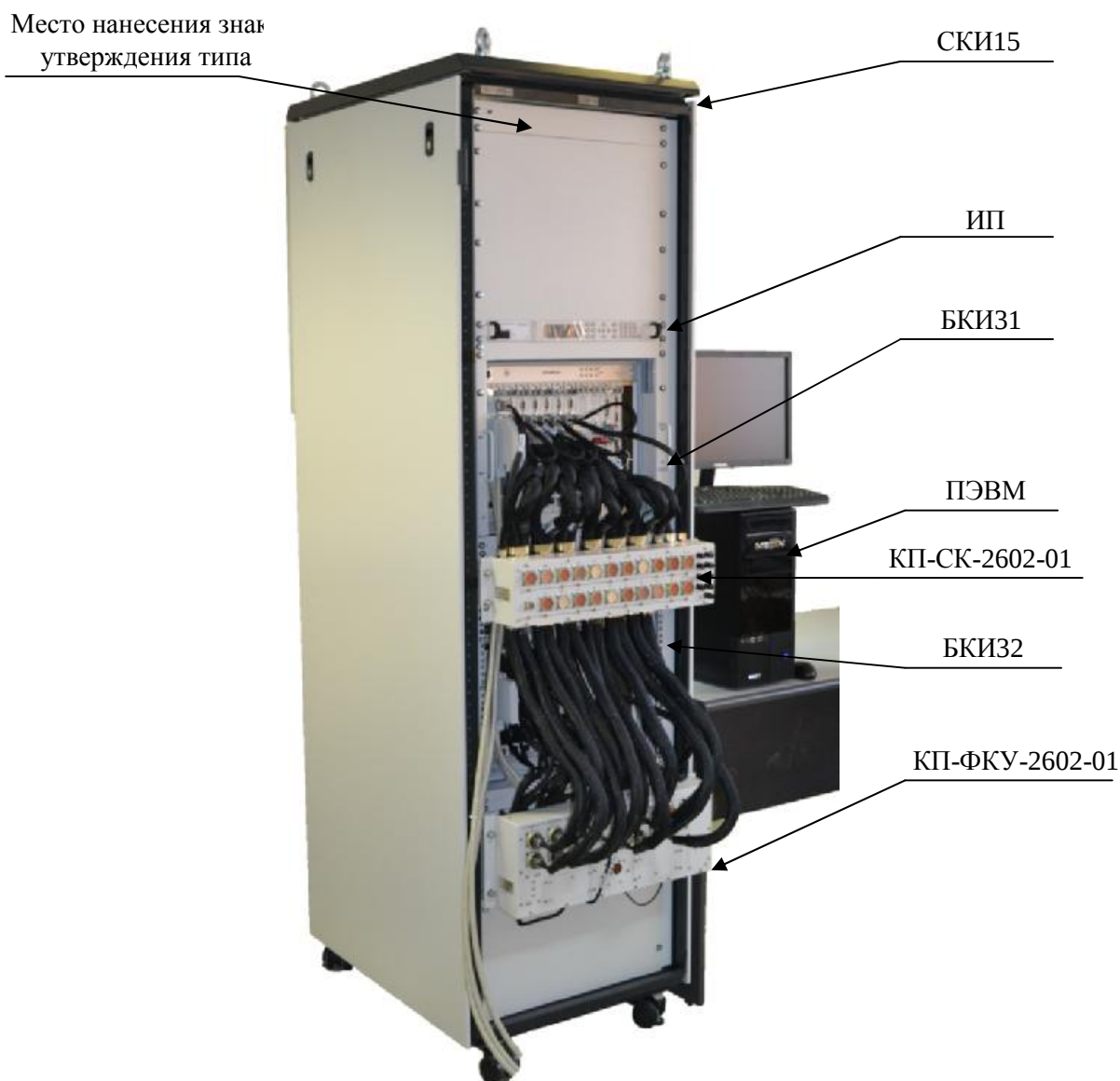
Рисунок 1 – Внешний вид системы ТЕСТ-2602-01 с указанием места нанесения знака утверждения типа
