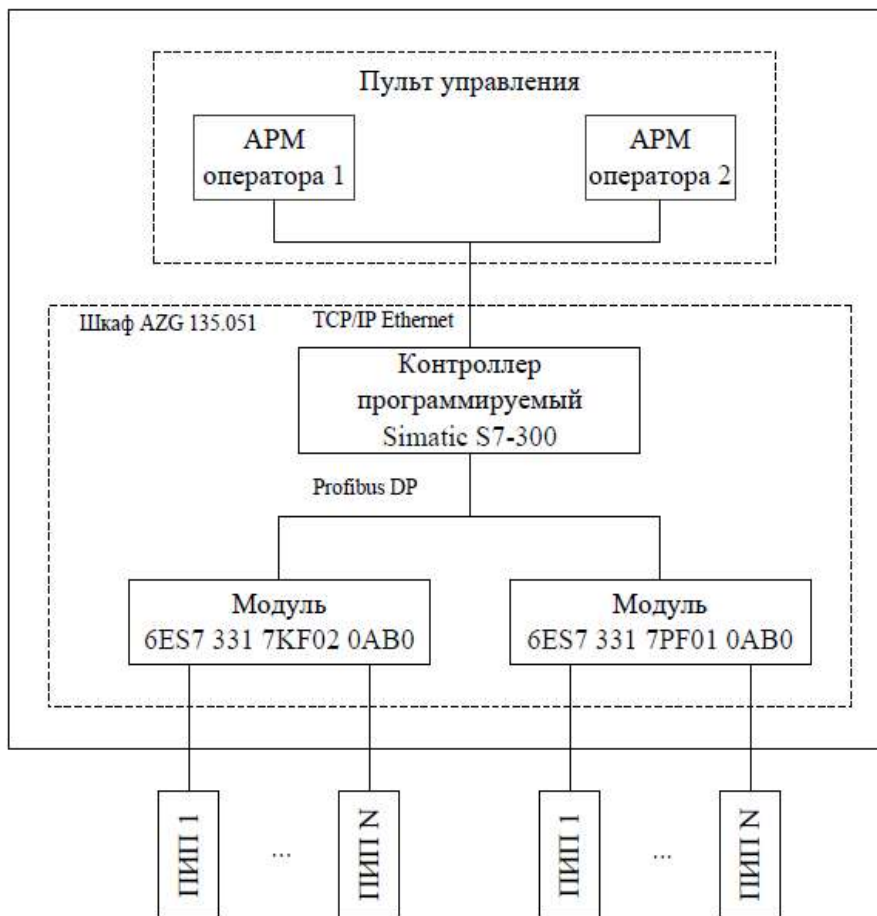
Рисунок 1 - Структурная схема ИУС
