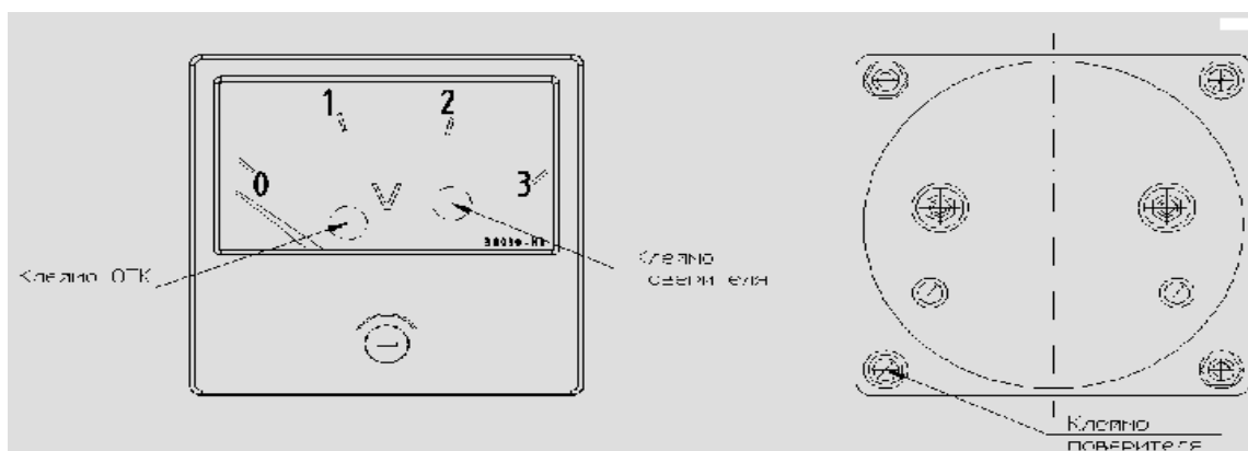
Рисунок 2 - Схема клеймения амперметров и вольтметров Э8030-М1, знак поверки наносится в виде клейма на прибор
