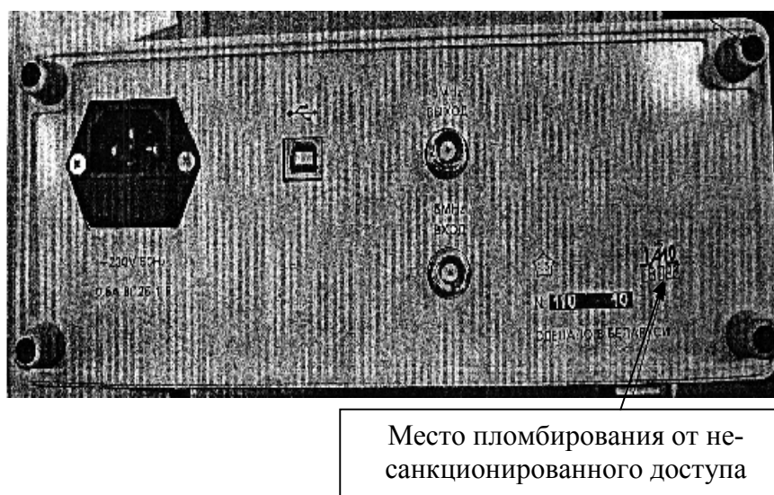
Рисунок 2 - Задняя панель частотомера
