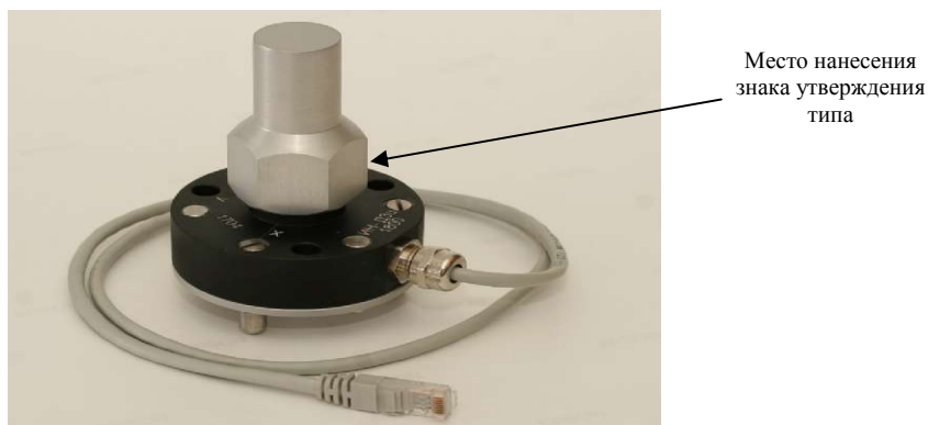
Рисунок 1 - Общий вид измерителя угла наклона двухкоординатного ИН-Д7 с цифровым выходом
