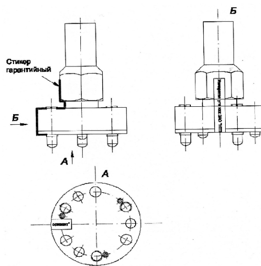
Рисунок 3 - Места пломбировки измерителя угла наклона двухкоординатного ИН-Д7
