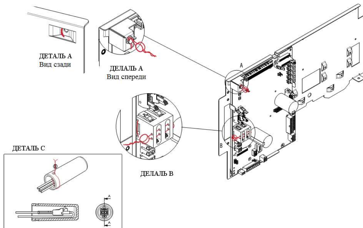
Рисунок 4 - Схема нанесения знака поверки на электронный блок
