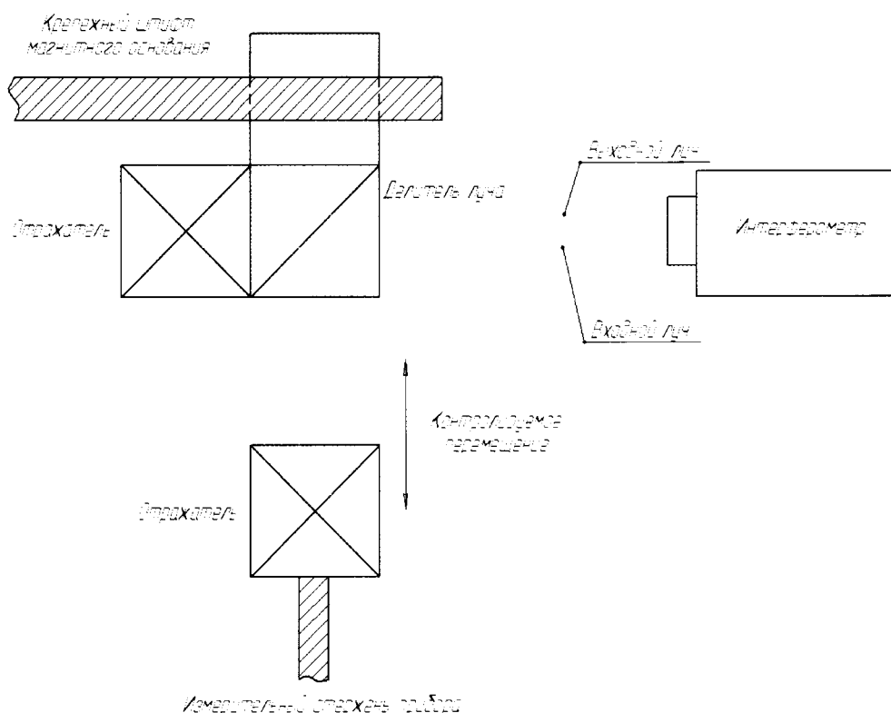
Рисунок 1. Схема установки оптических элементов и лазерной измерительной системы при поверке в вертикальном положении (вид сбоку)
