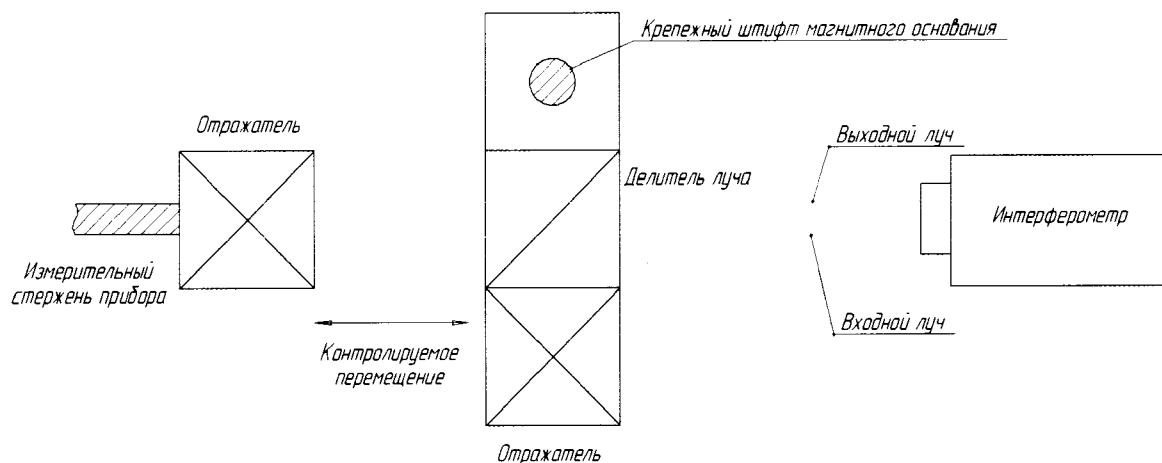
Рисунок 2. Схема установки оптических элементов и лазерной измерительной системы при поверке в горизонтальном положении (вид сверху)
