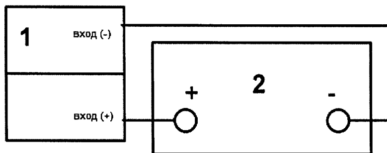
1 – модуль аналогового ввода; 2 – multifunctional калибратор; Рисунок А.2 – Схема соединения приборов при поверке входных/выходных аналоговых измерительных каналов типа «4 – 20 мА униполярный»
