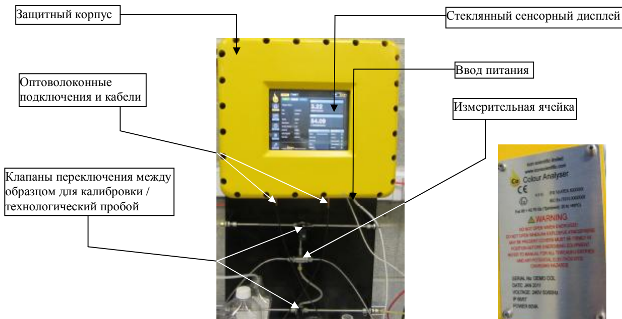
Рисунок 1. Внешний вид анализатора и его маркировка.
