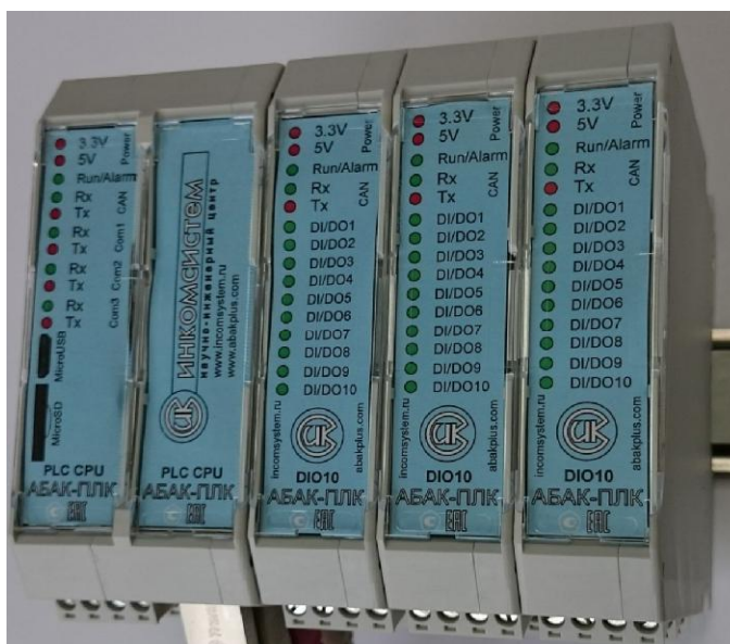
Рисунок 2 – Общий вид АБАК ПЛК в корпусе для установки на стандартную DIN-рейку
