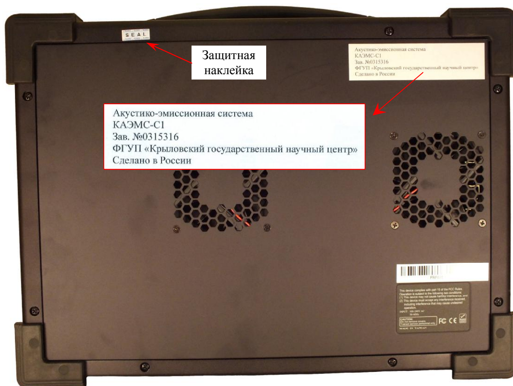
Рисунок 3 - Внешний вид модуля КАЭМС-С1 со стороны задней панели
