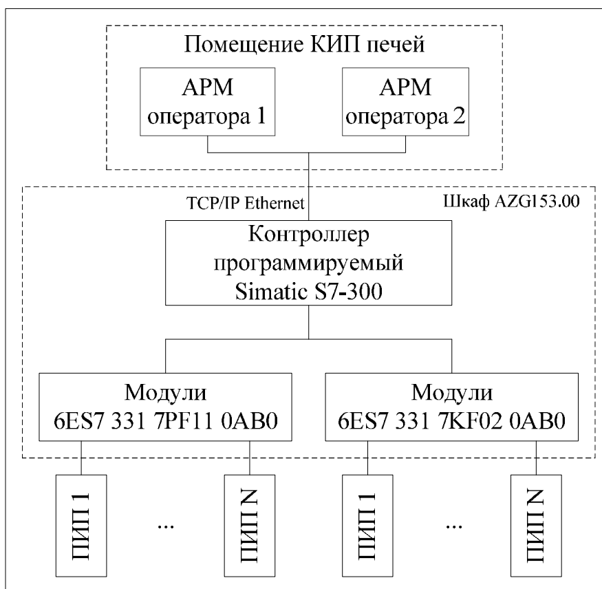
Рисунок 1 - Структурная схема ИУС
