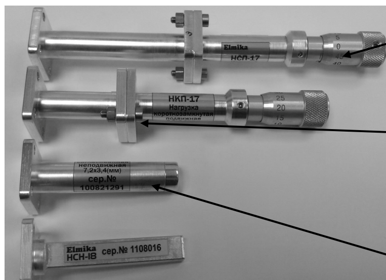
Рисунок 2- Схема пломбировки от несанкционированного доступа, обозначение мест нанесения знака утверждения типа и знака поверки
