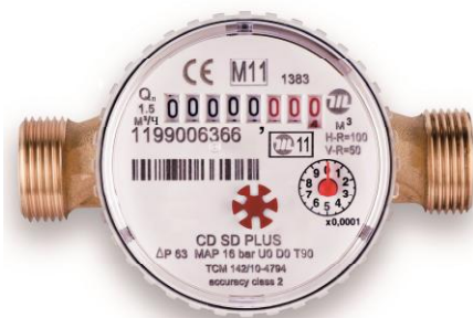
Рисунок 1 - Общий вид CD SD PLUS
