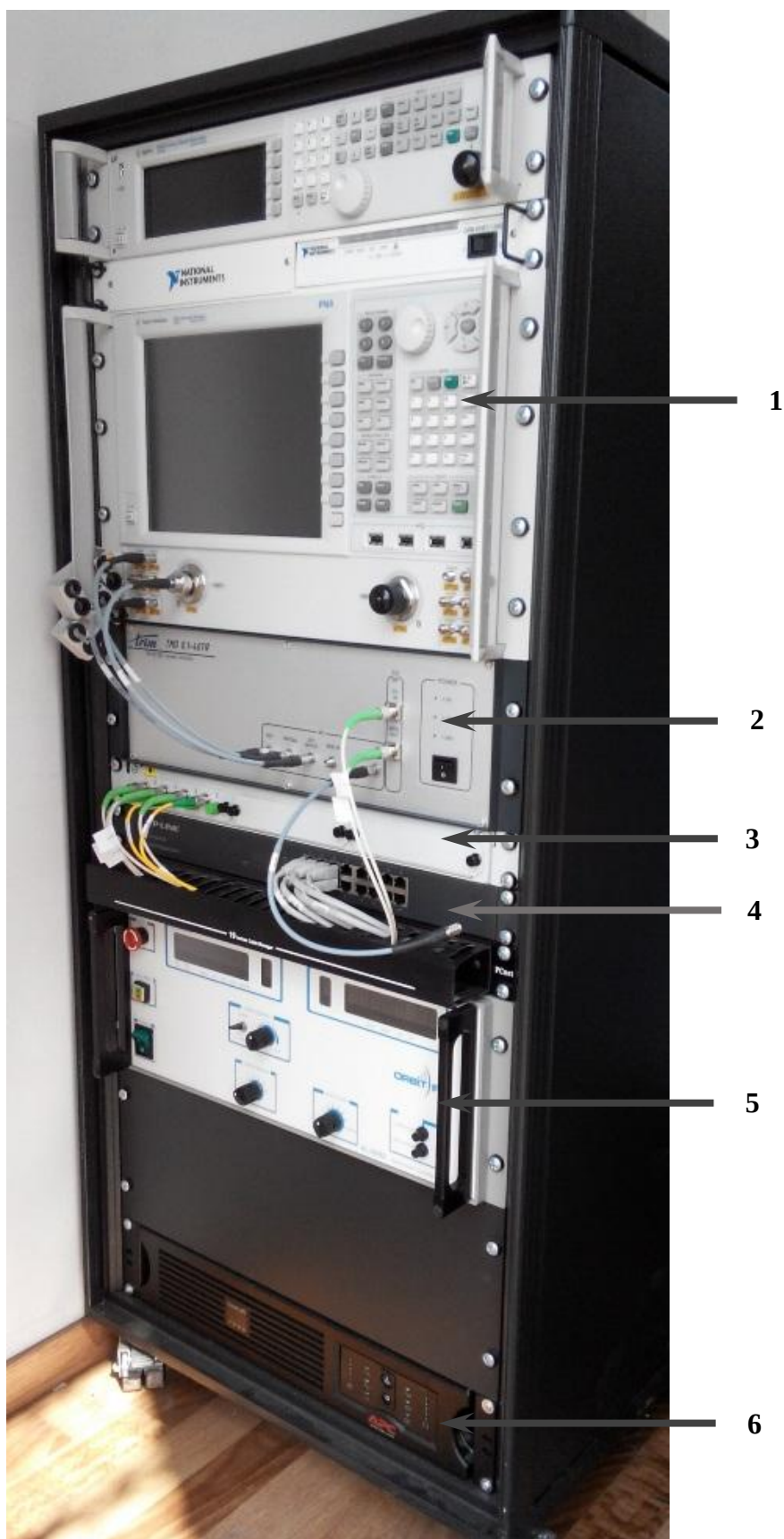
1 - ВАЦ N5224A, 2 - системный контроллер ТМО 0.1-40 TR, 3 - оптический бокс, 4 - сетевой коммутатор, 5 - контроллер перемещения AL-48062, 6 - источник бесперебойного питания
