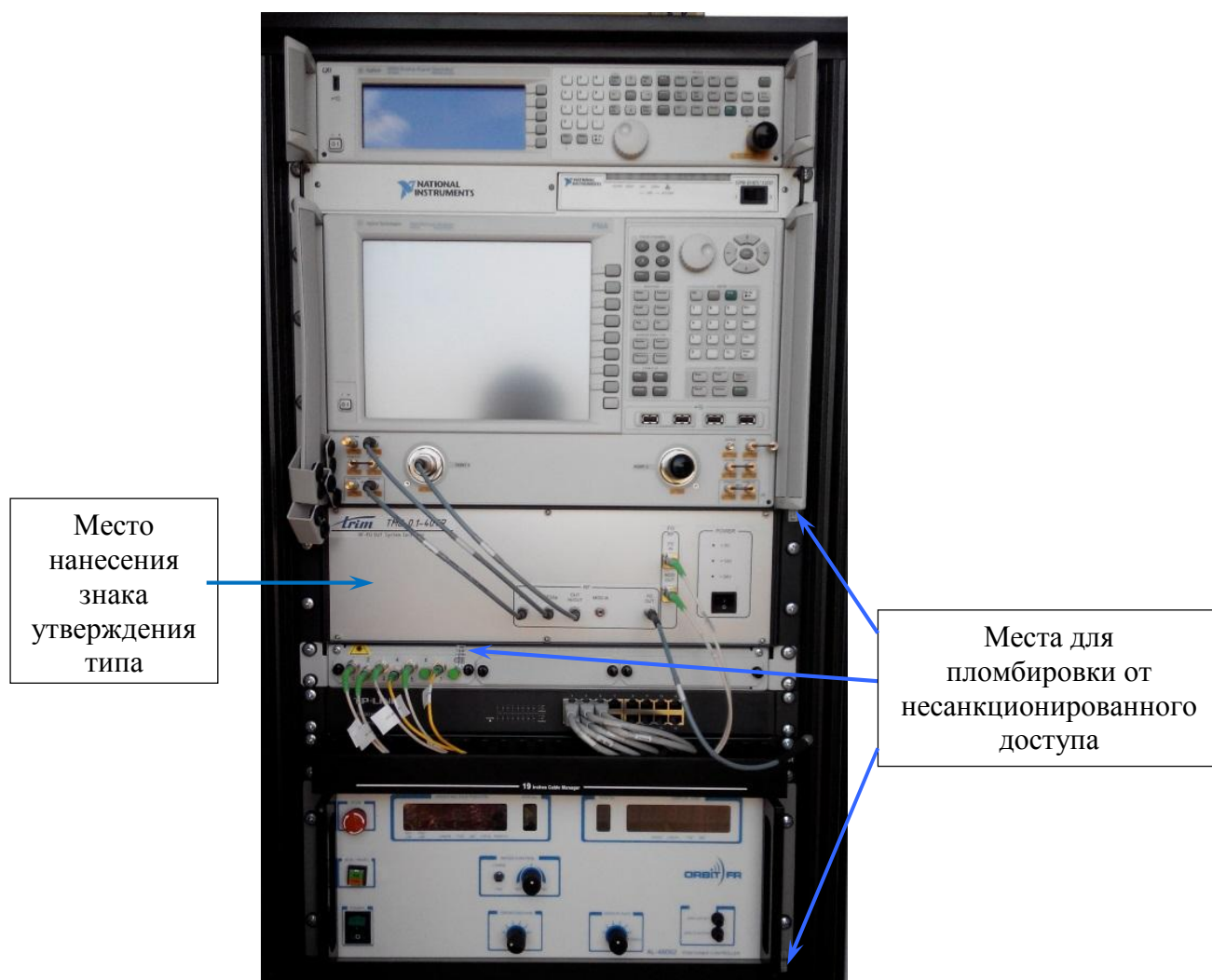
Рисунок 9 - Места пломбировки от несанкционированного доступа и размещения наклейки
