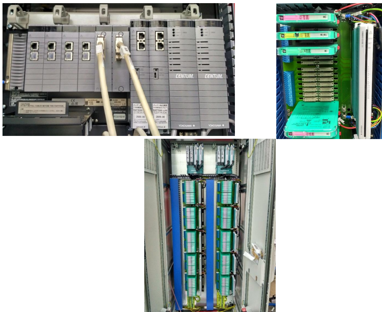
Рисунок 1 - Общий вид ИВК
