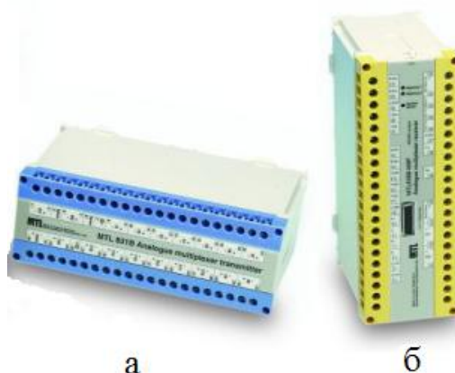
Рисунок 1 - Общий вид преобразователей измерительных многоканальных MTL830
