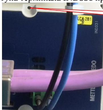
Рисунок 7 - Схема пломбировки от несанкционированного доступа терминала IND331
