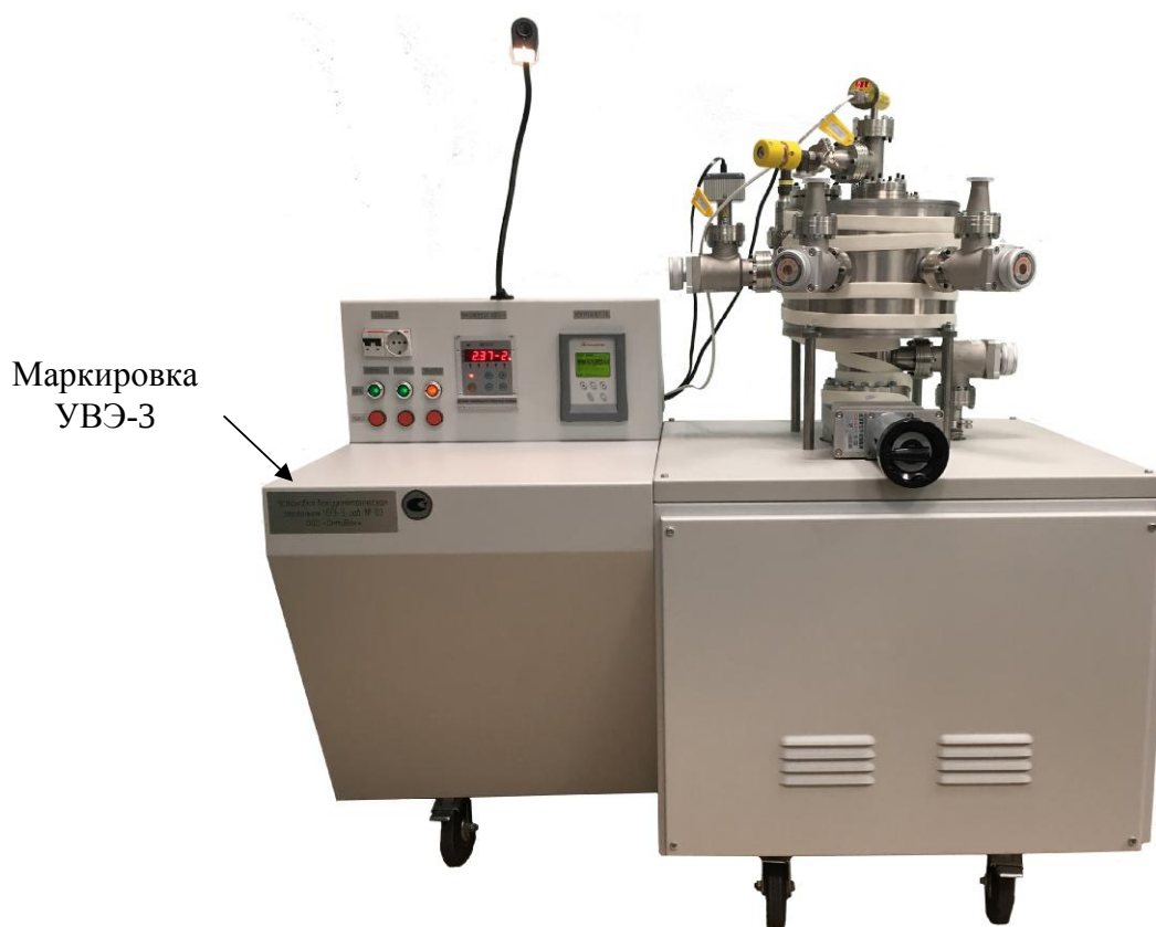
Рисунок 1 - Установка вакуумметрическая эталонная 2-го разряда УВЭ-3
