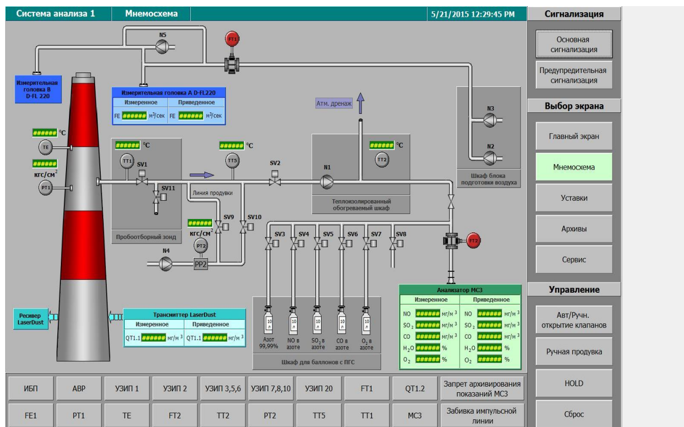
Рисунок 5 - Внешний вид мнемосхемы на дисплее АРМ системы
