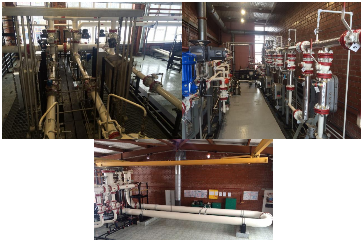
Рисунок 1 - Общий вид СИКН
