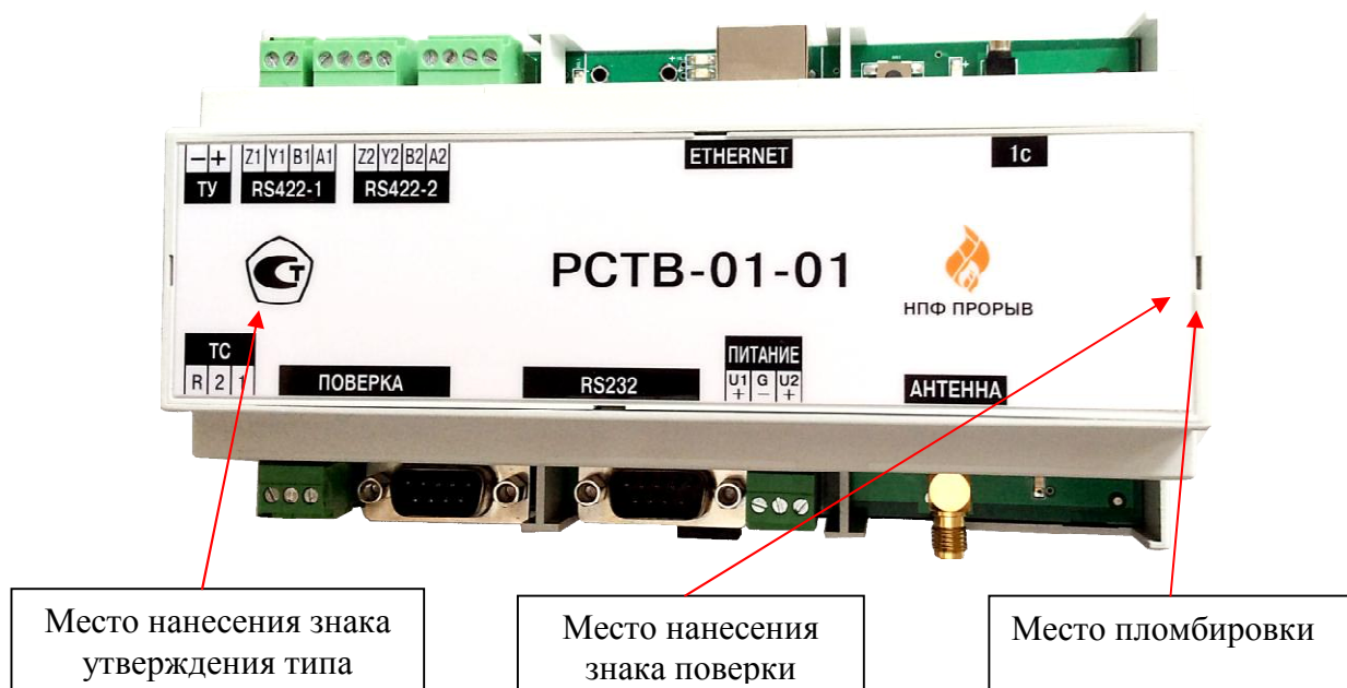
Рисунок 1 - Внешний вид РСТВ-01-01
