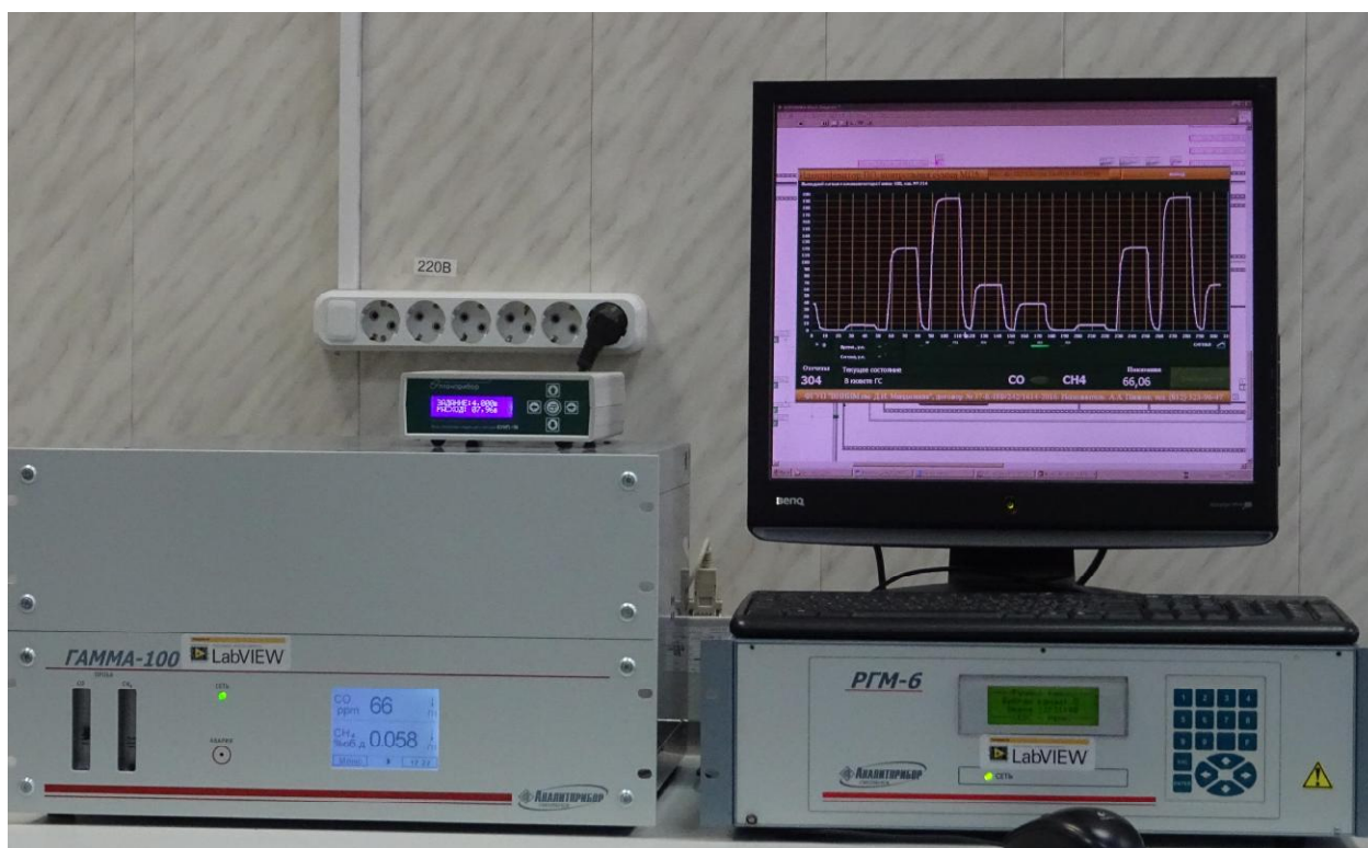
Рисунок 1 – Общий вид комплекса аппаратно-программного на базе газоанализатора ГАММА-100
