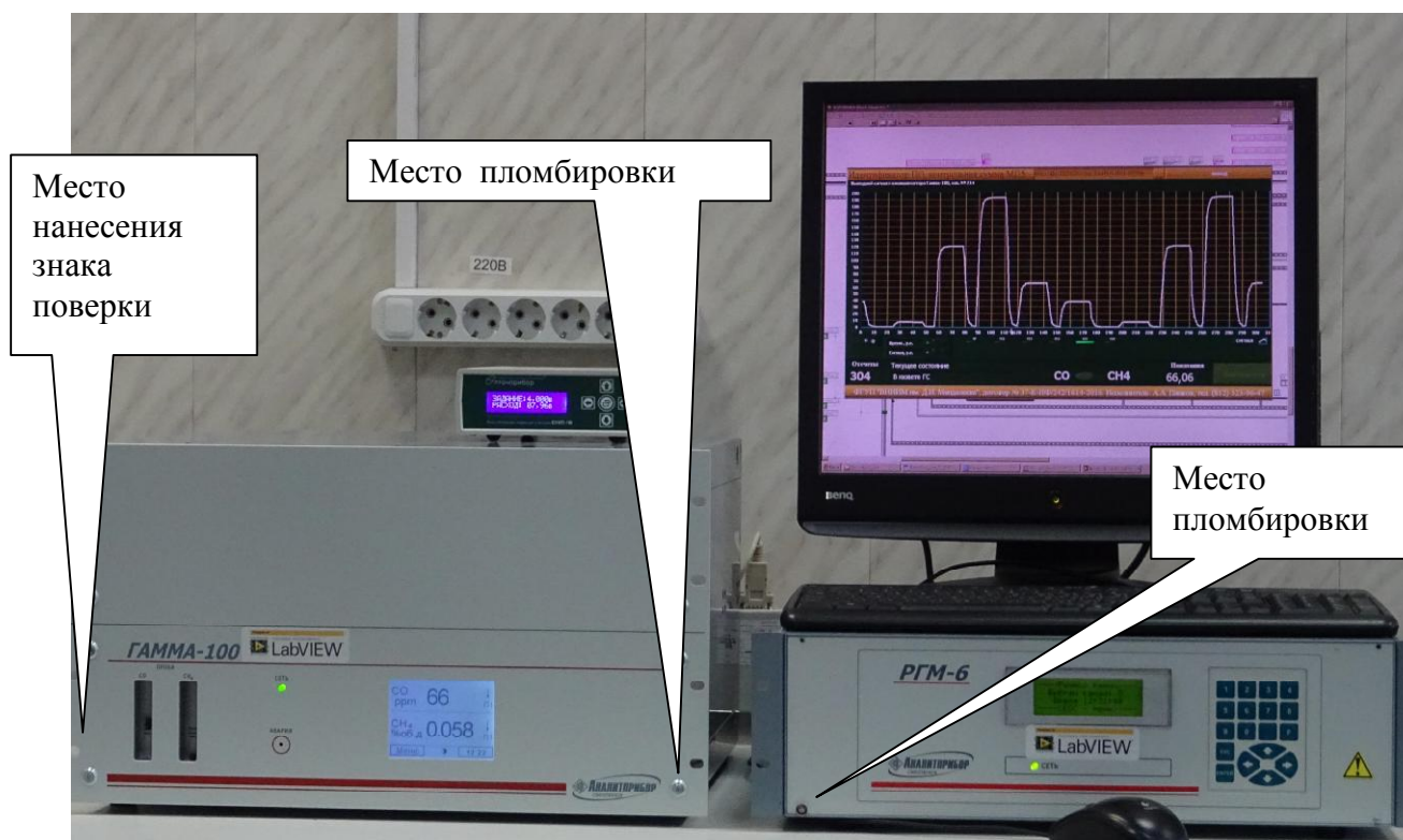
Рисунок 2 – Схема пломбировки от несанкционированного доступа и обозначение места нанесения поверки комплекса аппаратно-программного на базе газоанализатора ГАММА-100
