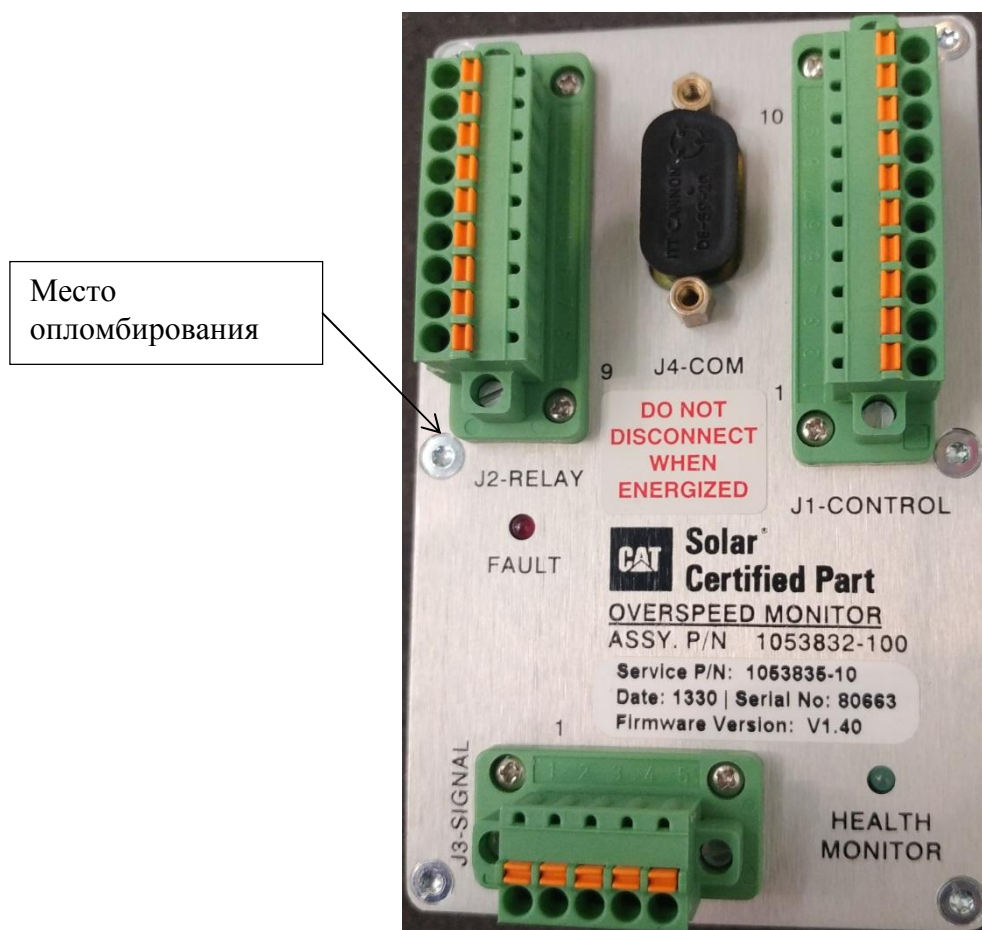
Рисунок 1 - Общий вид приборов для измерения частоты вращения Overspeed Monitor
