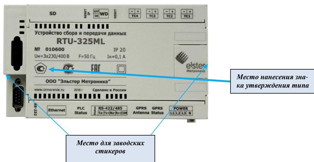
Рисунок 1 – Внешний вид средства измерений, схема пломбировки от несанкционированного доступа и обозначение места нанесения Знака утверждения типа
