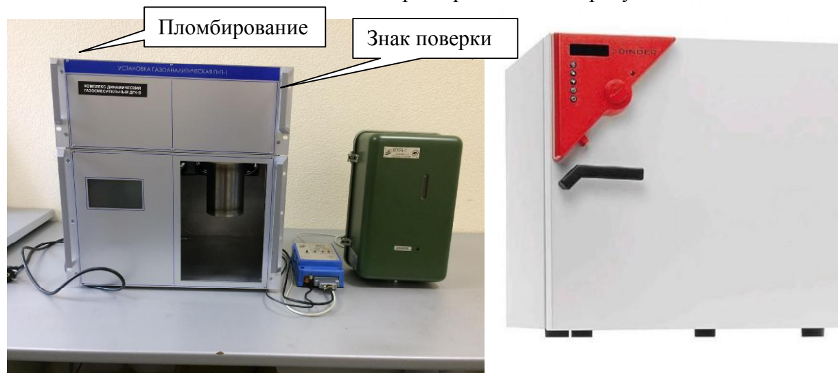
Рисунок 1 - Общий вид комплекса газоаналитического ГНП-1 (слева направо): установка ГНП-У1, аналитический блок, термошкаф Binder.
