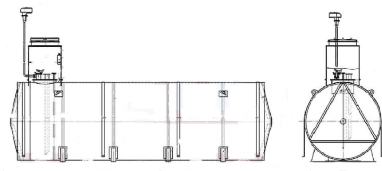
Рисунок 1 – Общий вид резервуара РГСД-50
