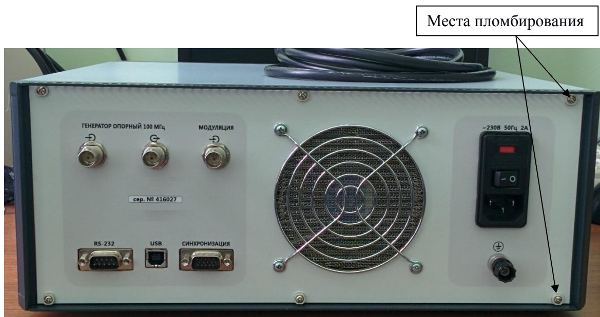
Рисунок 2 - Генератор Г4-MBM-118. Задняя панель
