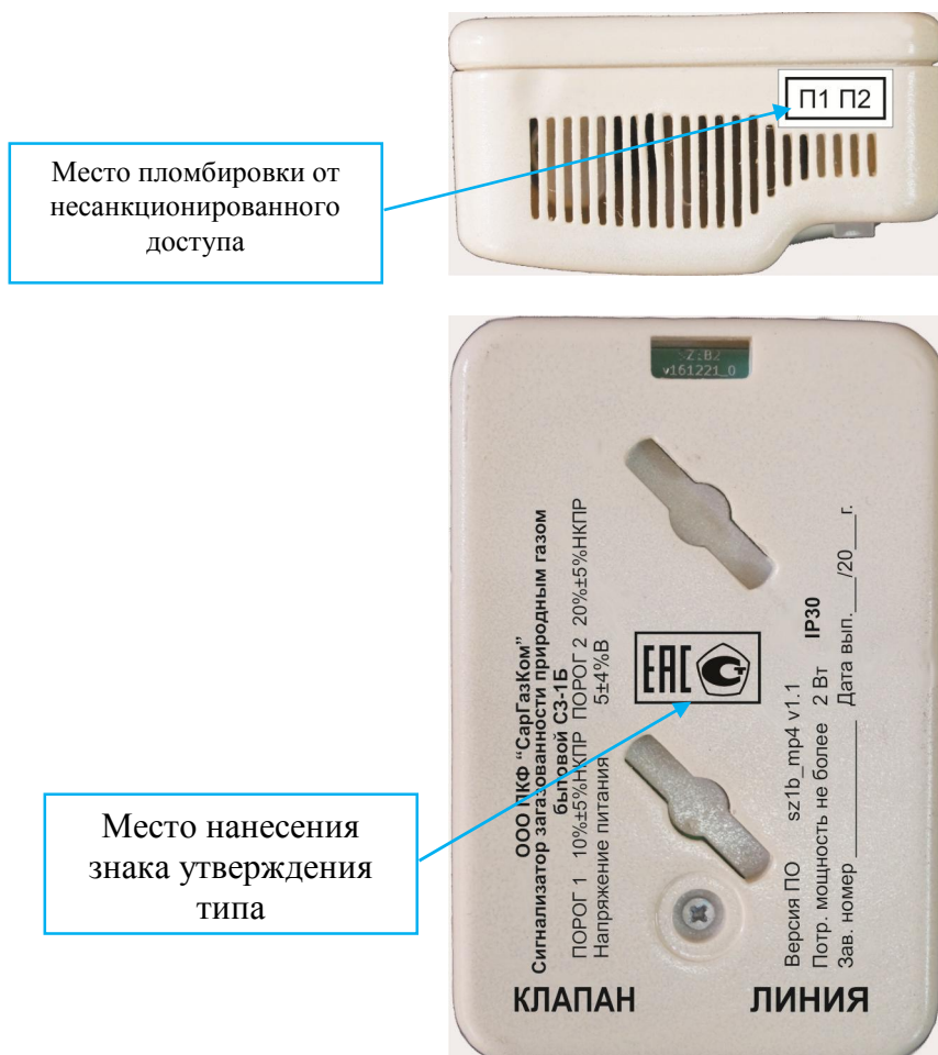
Рисунок 2 - Сигнализаторы загазованности бытовые СЗ-Б, место нанесения знака утверждения типа и пломбировки от несанкционированного доступа
