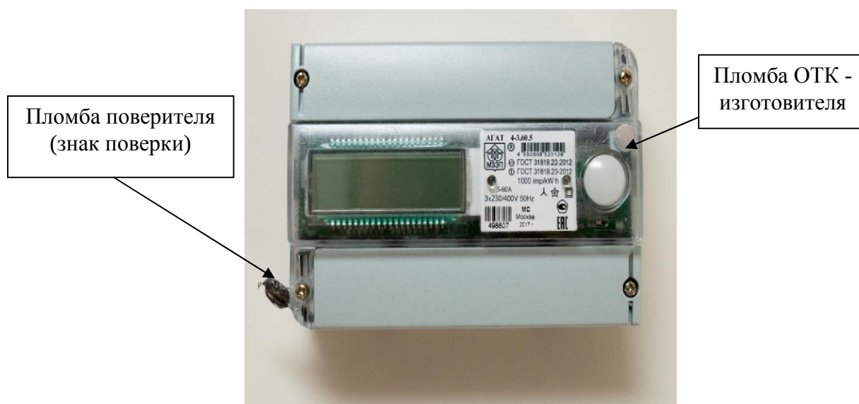
Рисунок 2 - Общий вид счетчиков в корпусе КЗ, схема пломбировки от несанкционированного доступа и обозначение места нанесения знака поверки
