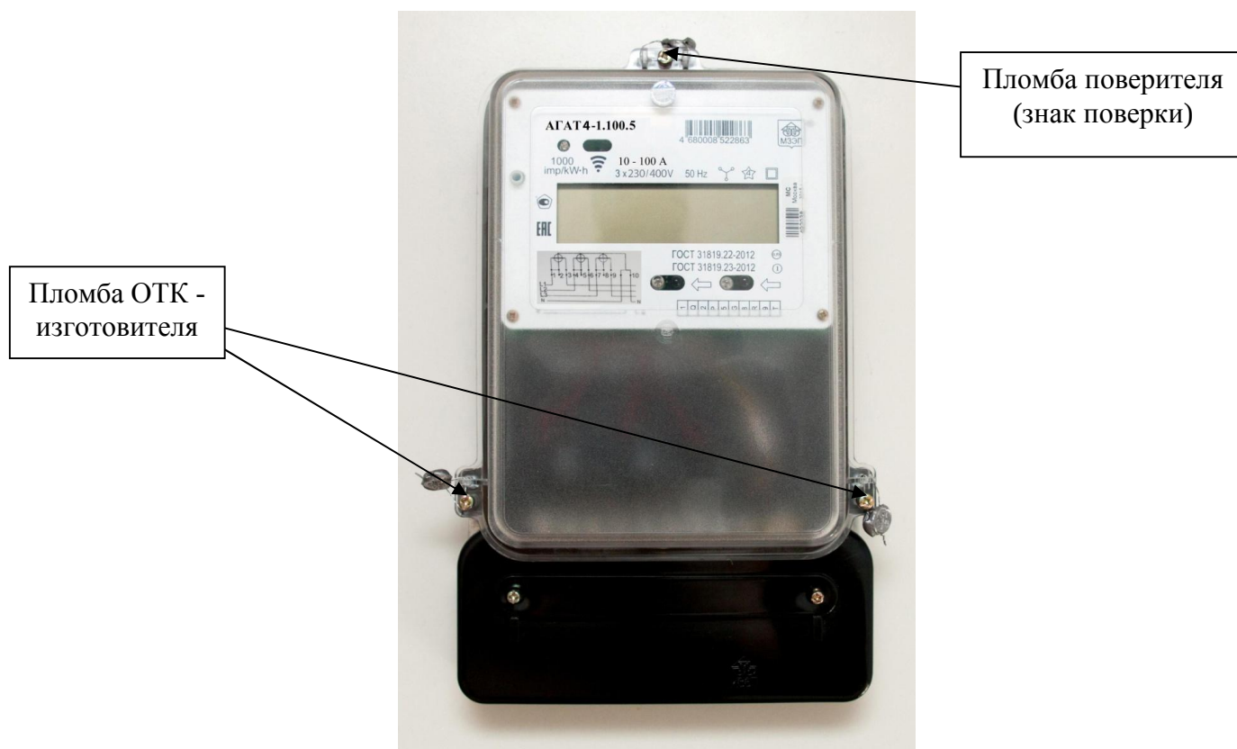
Рисунок 1 - Общий вид счетчиков в корпусе K1, схема пломбировки от несанкционированного доступа и обозначение места нанесения знака поверки
