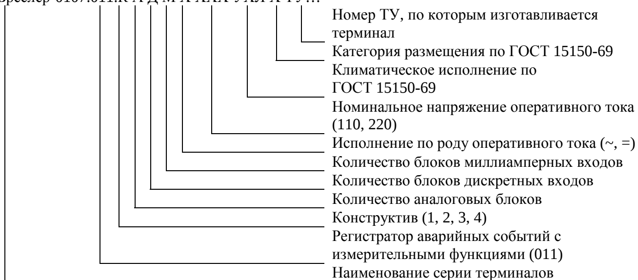
Рисунок 1 - Структура условного обозначения терминалов
