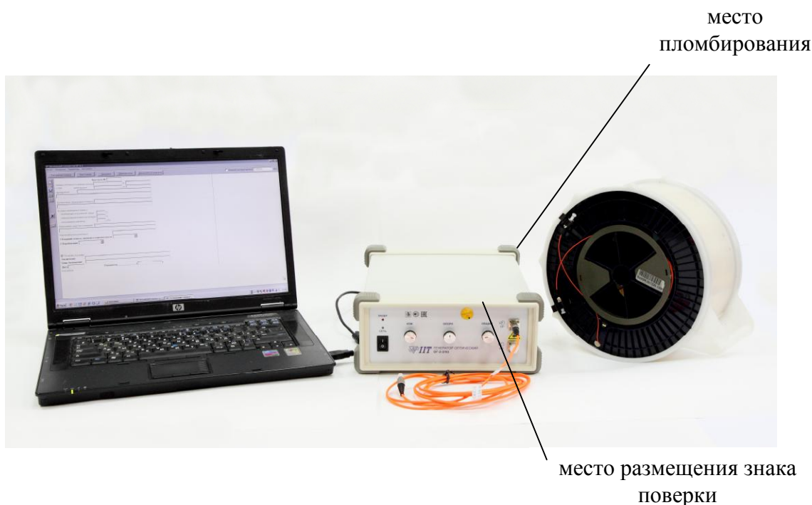
Рисунок 1 – Общий вид рабочего эталона единиц длины и ослабления в световоде РЭДО
