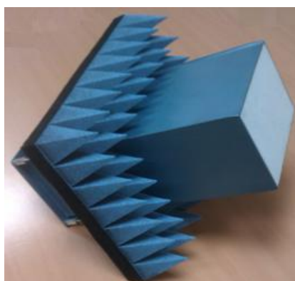
Рисунок 5 – Внешний вид антенн-зондов диапазона частот от 1 до 4 ГГц
