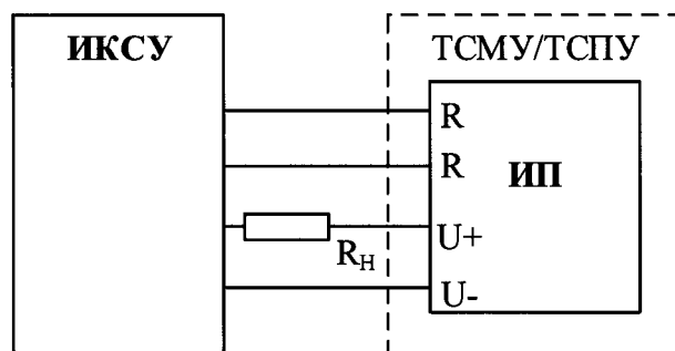
Рисунок 6.1 – Термопреобразователи с унифицированным выходным сигналом TCМУ-205-М, TCMY-205-Н, TCMY-205-МВ, ТСПУ-205-М, TCMY-205-Н, ТСПУ-205-МВ, ТСПУ-205Ex02. Схема электрическая соединений
