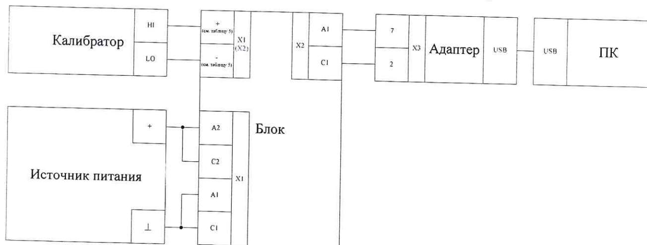
Рисунок А.1 – Схема подключения средств поверки к блоку
