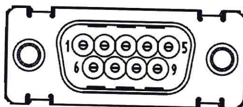
Рисунок Б.1 – Обозначение контактов адаптера
