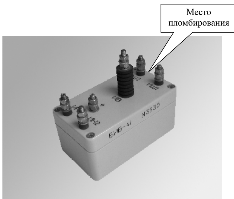
Общий вид блока измерения высоковольтного БИБ-41/41М
