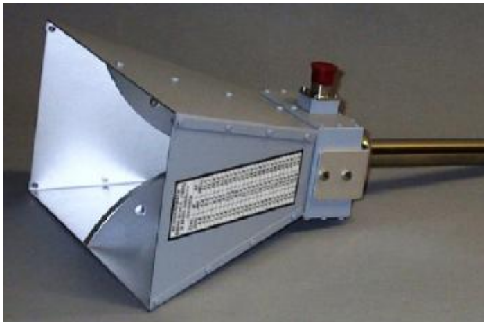
Рисунок 1 – Внешний вид рупора ВВНА 9120 А
