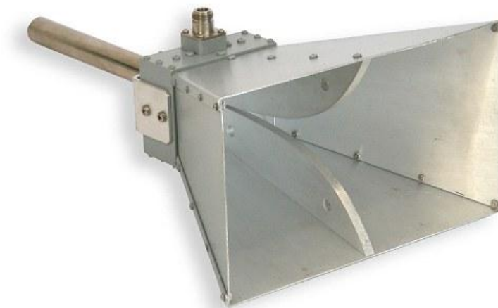
Рисунок 9 – Внешний вид рупора ВВНА 9120 L3F
