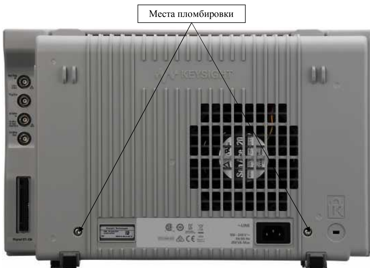
Рисунок 3 - Общий вид базового блока анализаторов SX3322A, SX3324A. Вид сзади. Схема пломбировки от несанкционированного доступа
