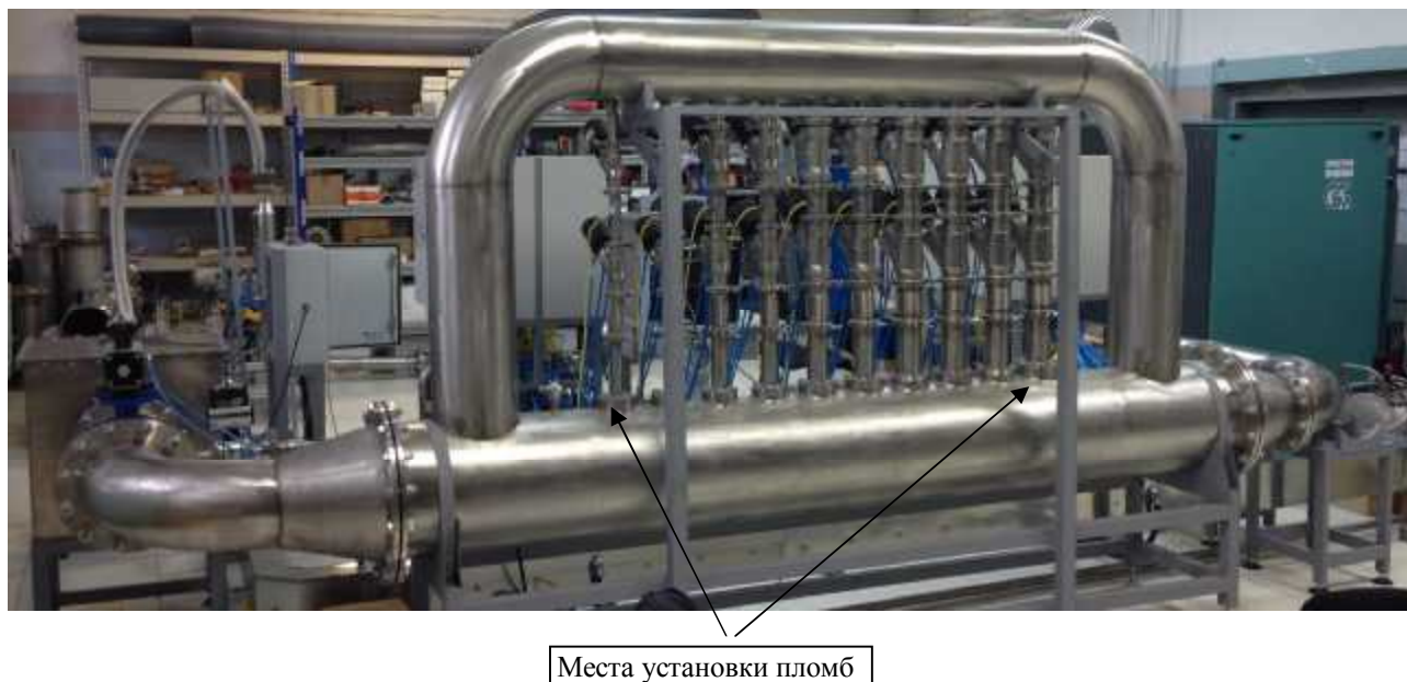
Рисунок 2 - Общий вид установки (большой сопловой блок)
