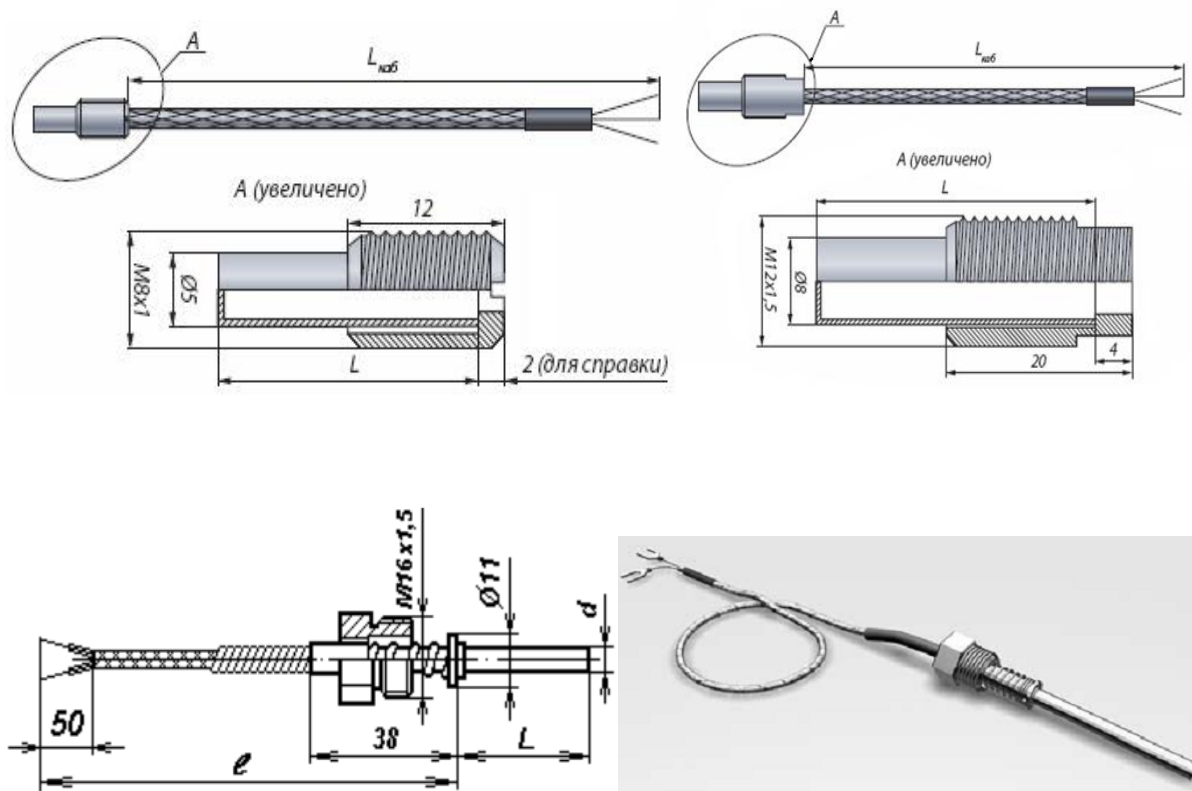
Рисунок 10 - Общий вид модификации КТ-110
