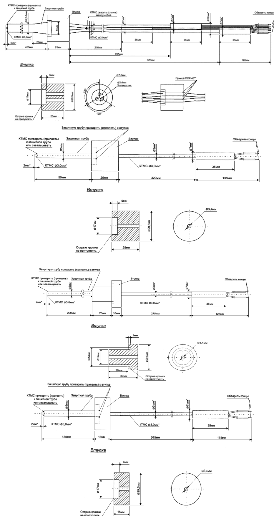
Рисунок 9 - Общий вид модификации КТ-109
