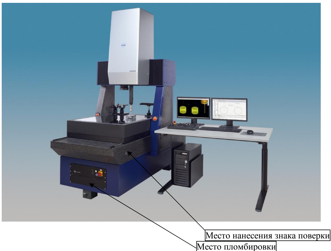
Рисунок 1 - Общий вид, схема пломбировки от несанкционированного доступа, обозначение места нанесения знака поверки машин моделей ScopeCheck FB DZ
