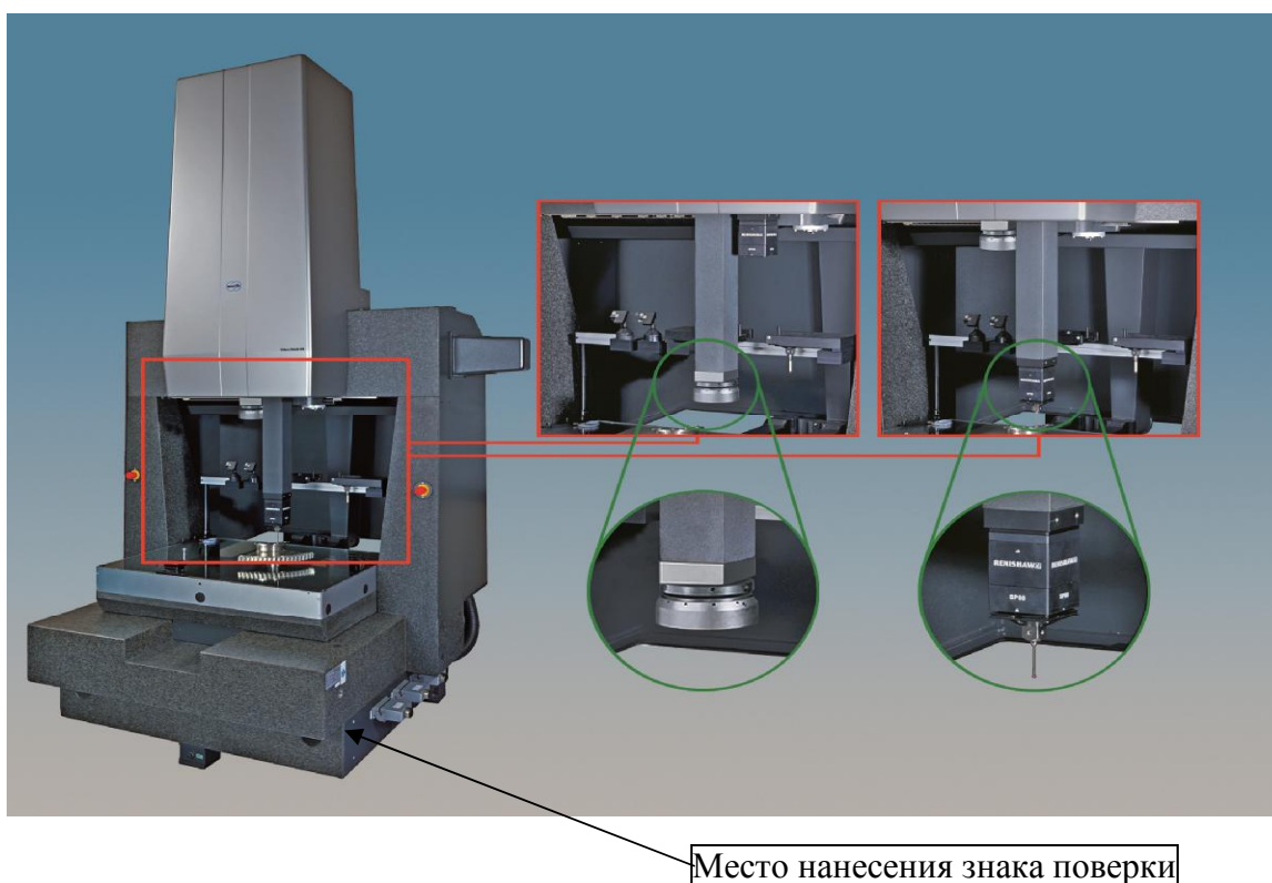
Рисунок 2 - Общий вид, обозначение места нанесения знака поверки машин моделей VideoCheck DZ, VideoCheck DZ HA
