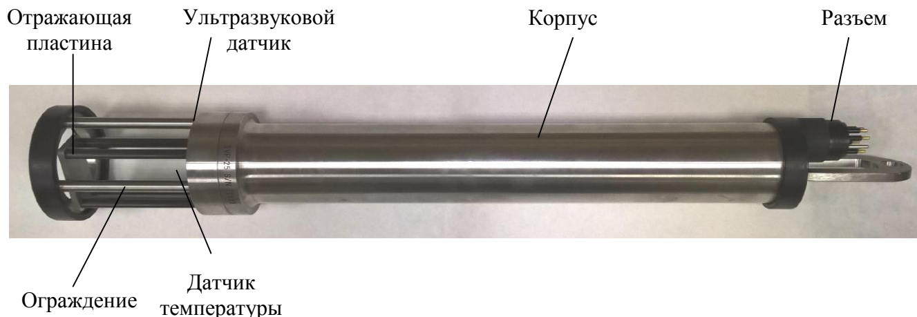
Рисунок 1 - Внешний вид зондов
