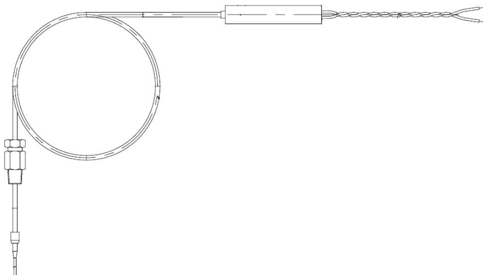
Рисунок 1 - Общий вид преобразователей термоэлектрических модели 381A6581
