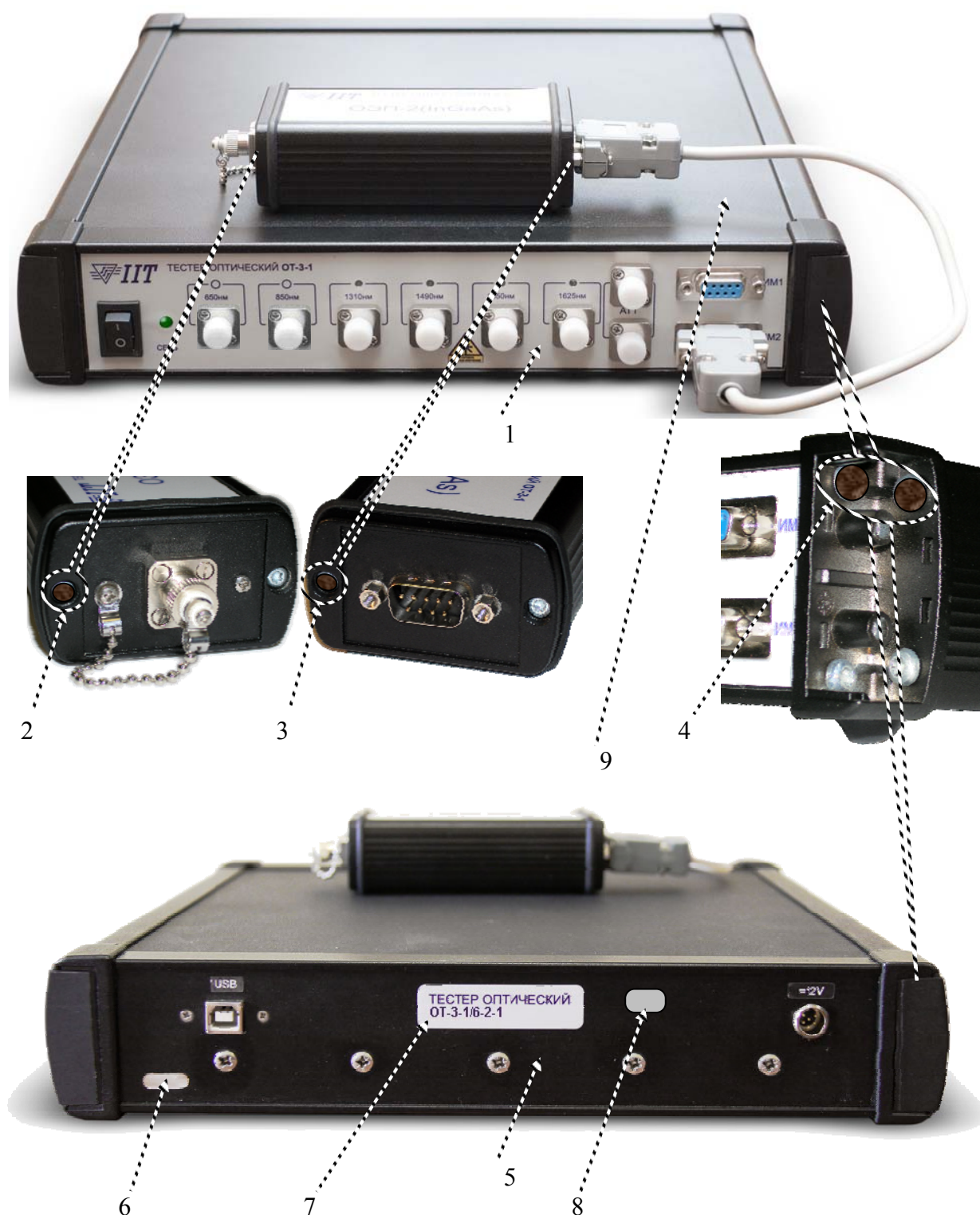
Рисунок 1 - Общий вид тестера, места пломбирования и маркировки
