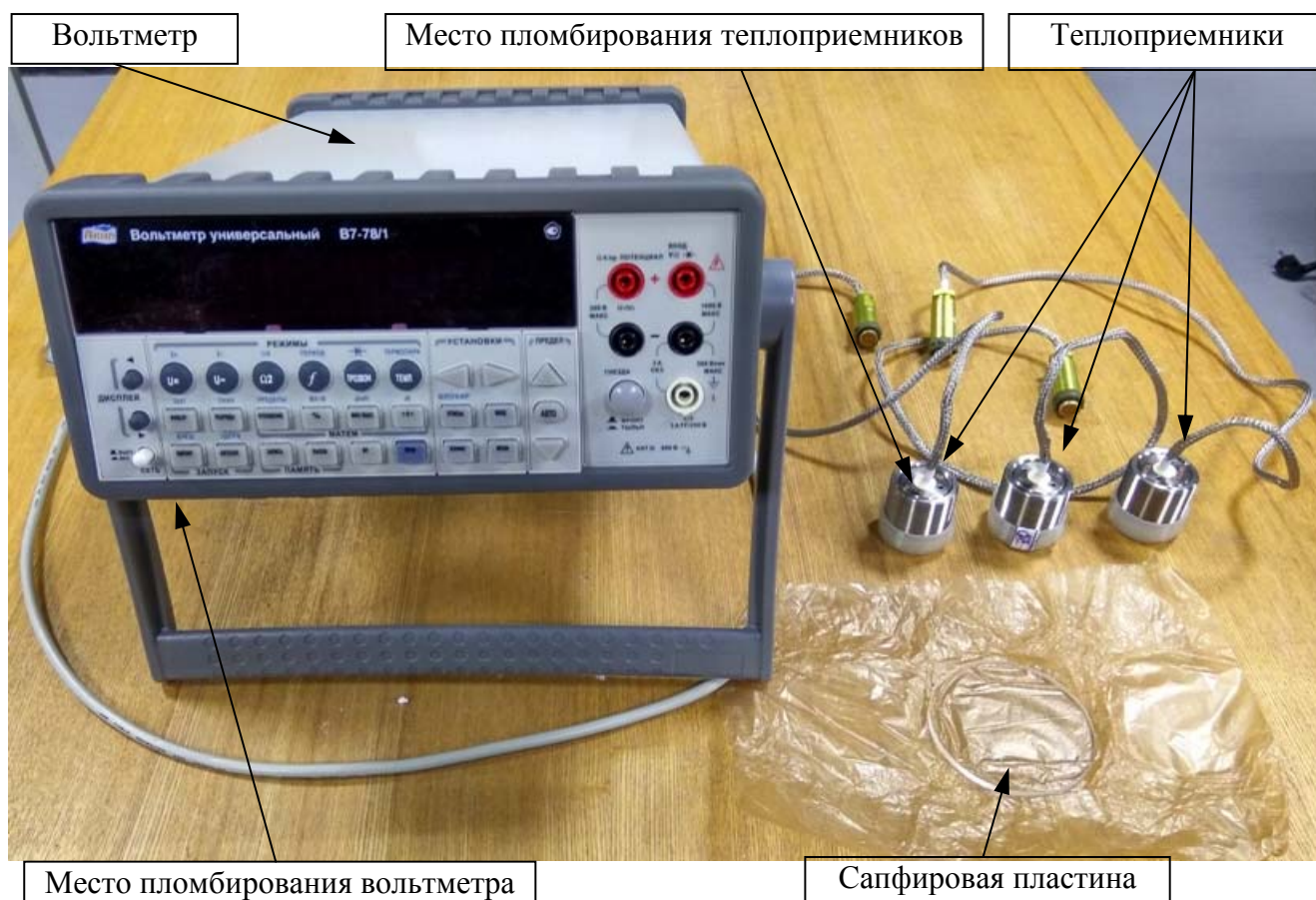
Рисунок 1 - Общий вид прецизионных радиометров со схемой пломбировки
