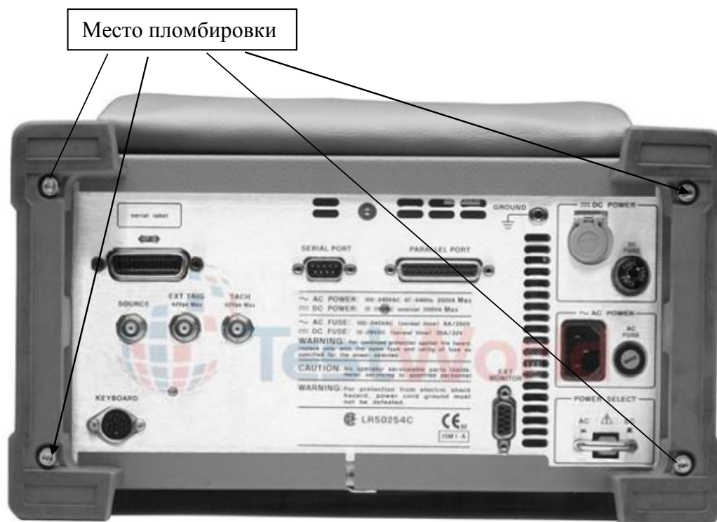
Рисунок 2 - Задняя панель анализатора. Места пломбировки от несанкционированного доступа
