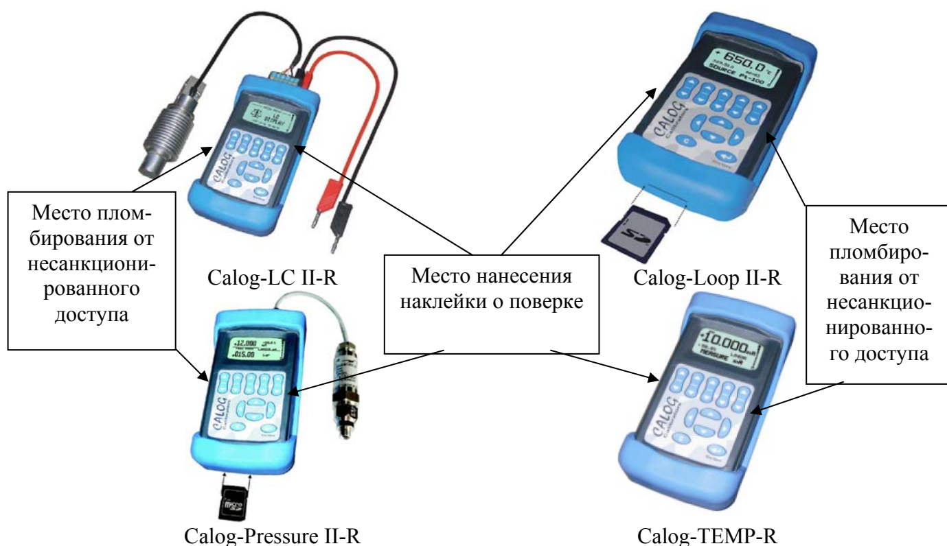
Рисунок 1 - Общий вид, места пломбирования и нанесения знака поверки
