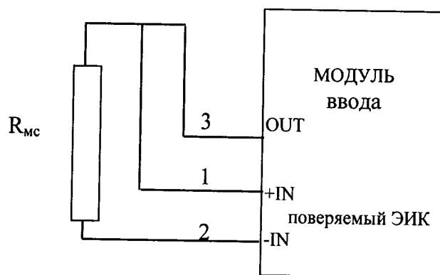
R_{мс} – магазин сопротивлений
