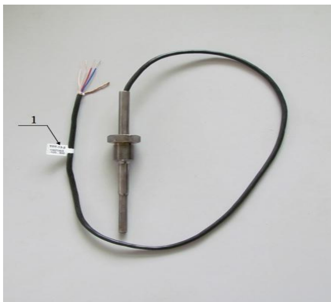
Рисунок 5 – Внешний вид термопреобразователей (1 – место нанесения маркировки)
